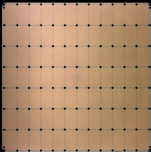
Cerebras WSE 2
